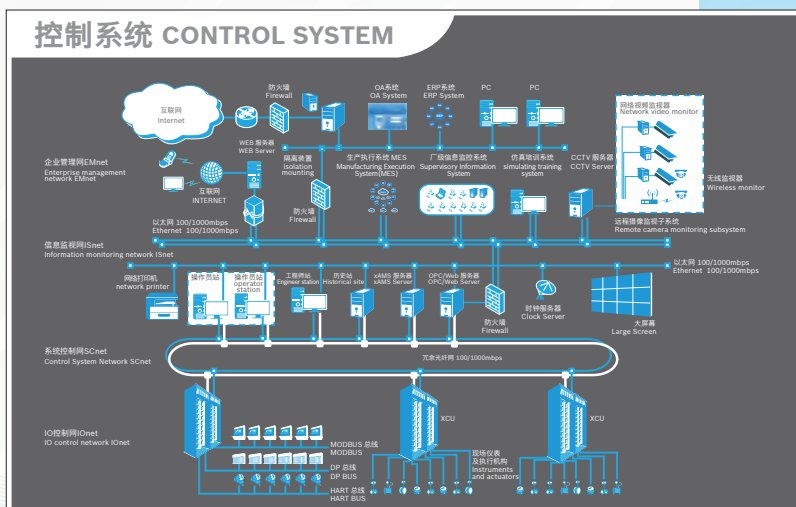
智能化数字工厂控制系统拓扑图
