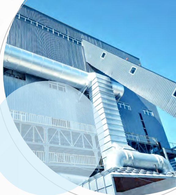
矿热炉外貌
